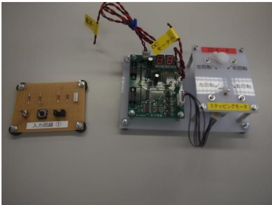
課題使用機器（左側が入力回路）
